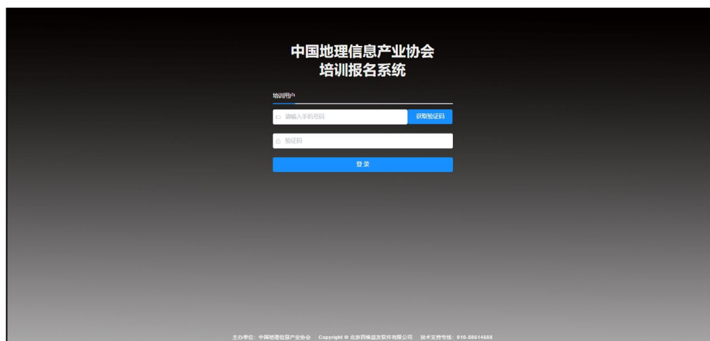
图 1 系统界面
